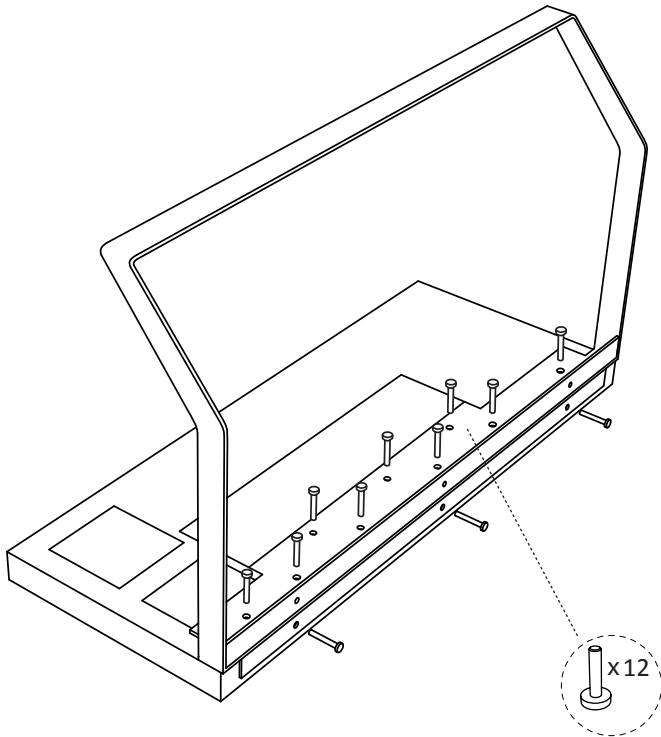
Montering af stel på bordplade
